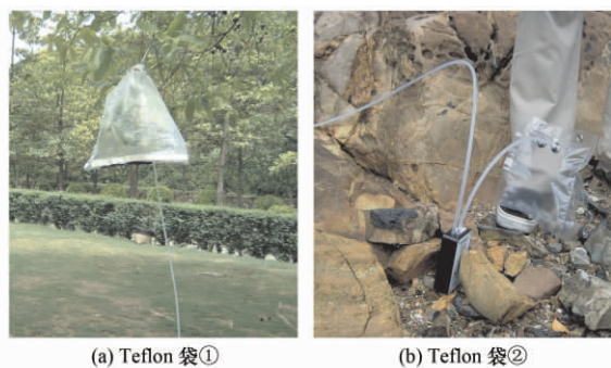
图 1 采集气体样品的 Teflon 袋 Fig. 1 Teflon sealed bags used for gas collection
