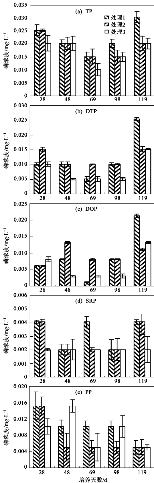
图2 不同处理上覆水磷形态浓度的变化
