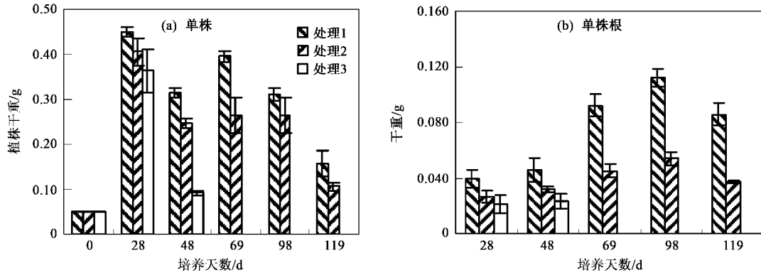
图3 沉水植物穗状狐尾藻生物量与根重随时间的变化曲线
