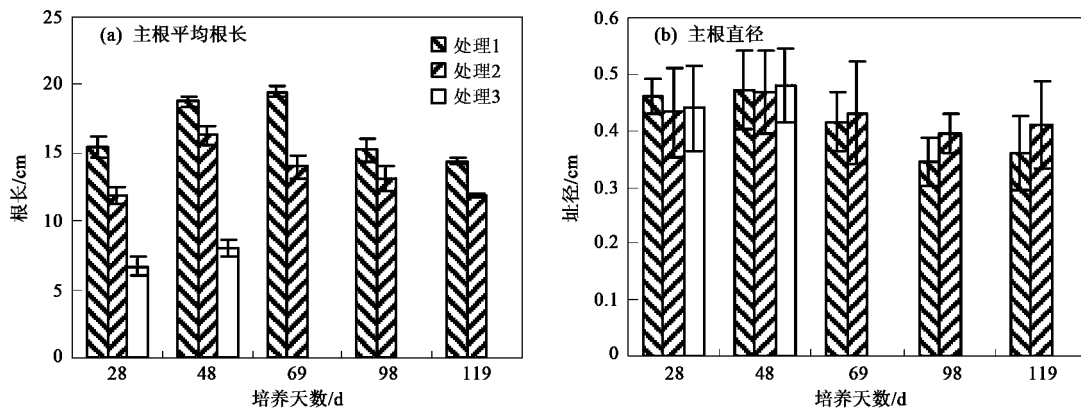
图4 沉水植物穗状狐尾藻主根平均根长和主根直径随时间的变化
