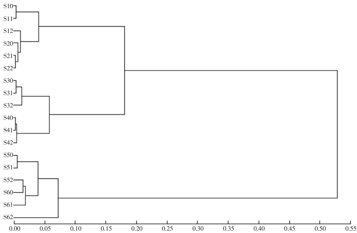
图 2 基于欧氏距离平方和离差平方方法的聚类分析树形图
