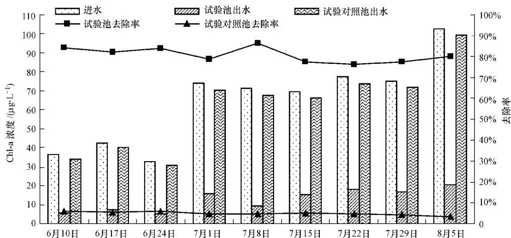
图 3 Chl-a 的去除效果
