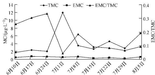
图 4 进水总藻毒素和胞外藻毒素的变化情况
