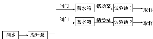
图 1 试验工艺图
