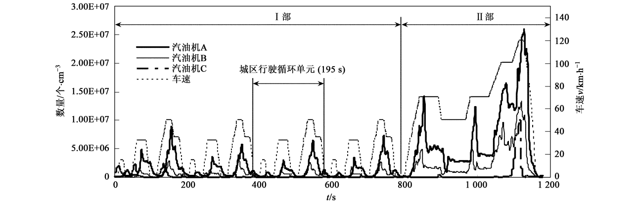
图 2 汽油车瞬态循环颗粒物排放
