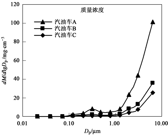
图 4 排气颗粒物质量浓度分布
