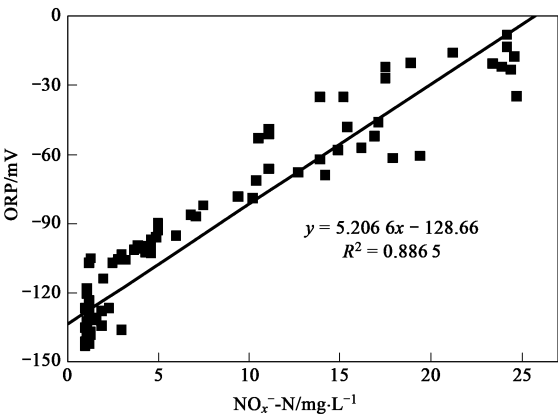
图2 硝酸盐氮与 ORP 的相关关系 Fig. 2 Relationship of nitrate and ORP value
