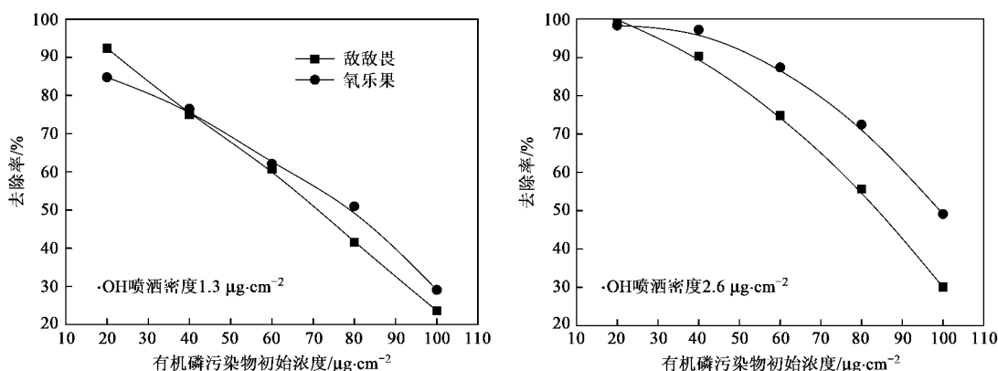
图 3 有机磷污染物初始密度对去除率的影响曲线
