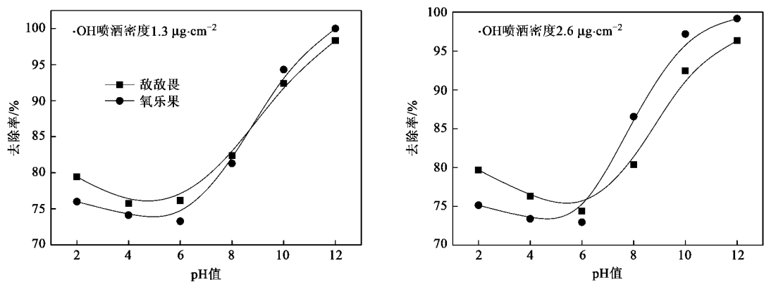
图 4 pH 值对表面有机磷污染物去除率的影响曲线 Fig. 4 Effects of pH value on the removal rate
