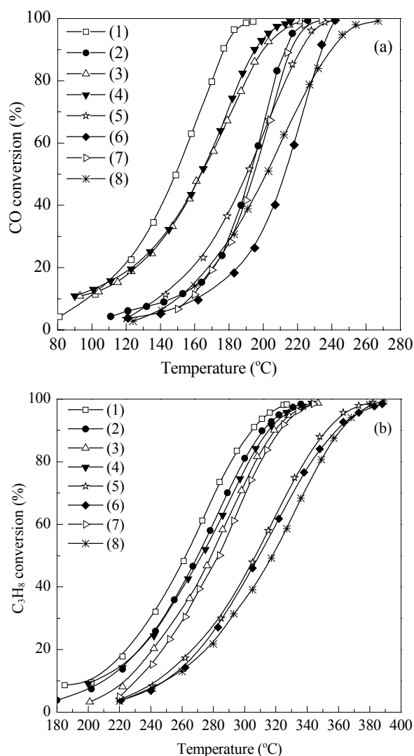
图 6 不同催化剂对 CO 和 \text{C}_3\text{H}_8 的催化氧化活性
