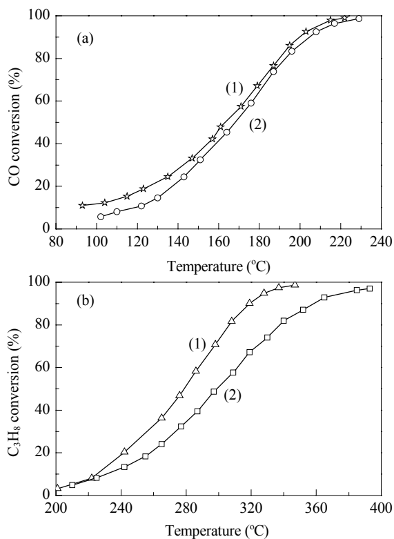
图 7 \text{Mn/LaCeZr/Al}_2\text{O}_3 -650 催化剂的抗硫性能
