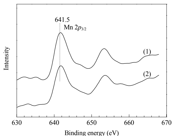
图 5 500 °C 焙烧的改性 \text{Al}_2\text{O}_3 负载的催化剂中 Mn 元素的 XPS 谱
