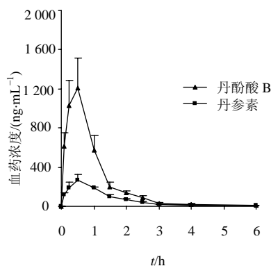
图 3 大鼠 ig 500 mg/kg 丹酚酸 B 后丹酚酸 B 和丹参素的平均血药浓度-时间曲线 ( \bar{x} \pm s, n = 6 ) Fig. 3 Mean plasma concentration-time profiles of SalB and DSS after ig Sal B to rats at a dose of 500 mg/kg ( \bar{x} \pm s, n = 6 )
