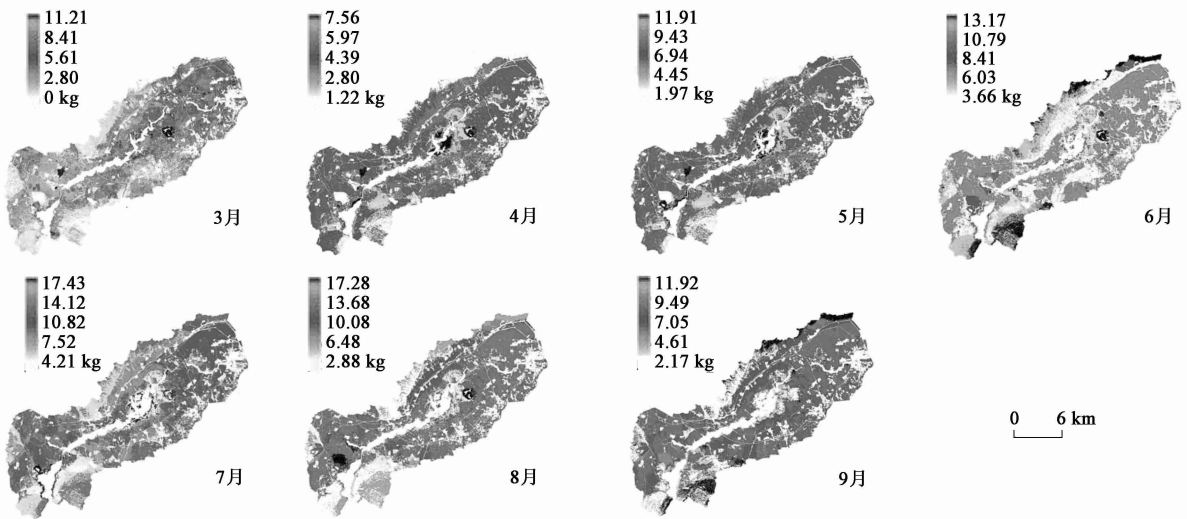
图 6 官厅水库库滨带流域对氮元素去除量空间分布
