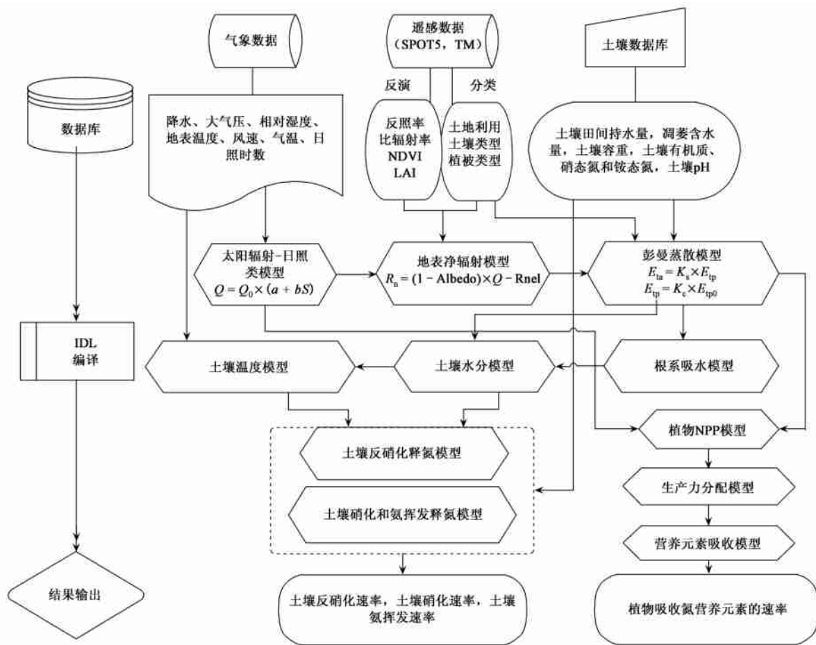
图 2 RIP_N 模型计算流程
