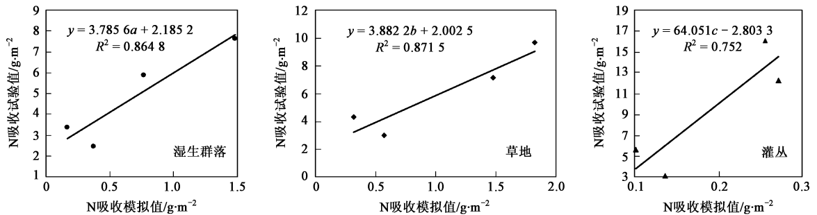
图 7 植物对氮元素吸收负荷的模拟值与试验值的相关分析
