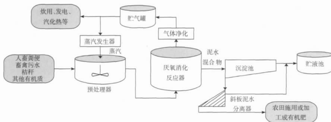
图 1 生物质厌氧消化系统
