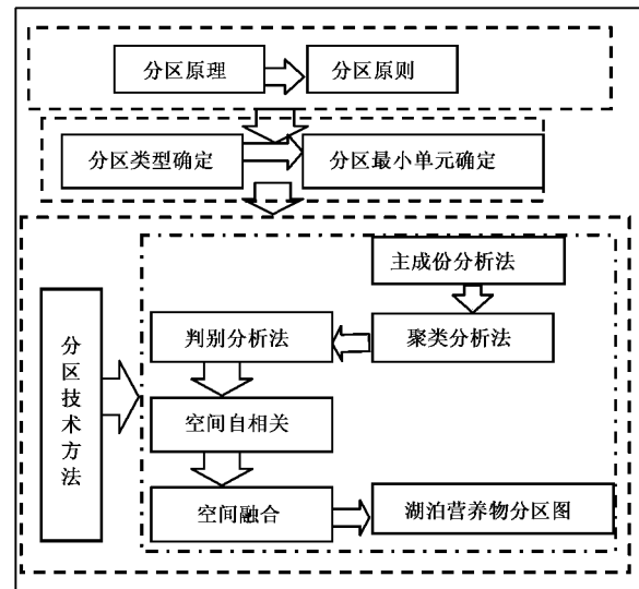
图 1 湖泊营养物生态分区技术方法
