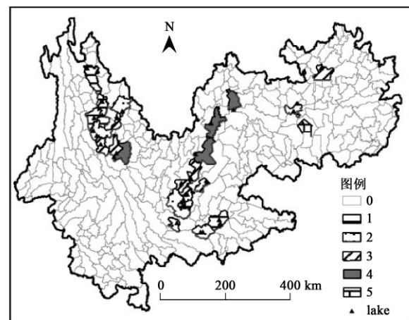
图 2 两步聚类湖泊流域分类
