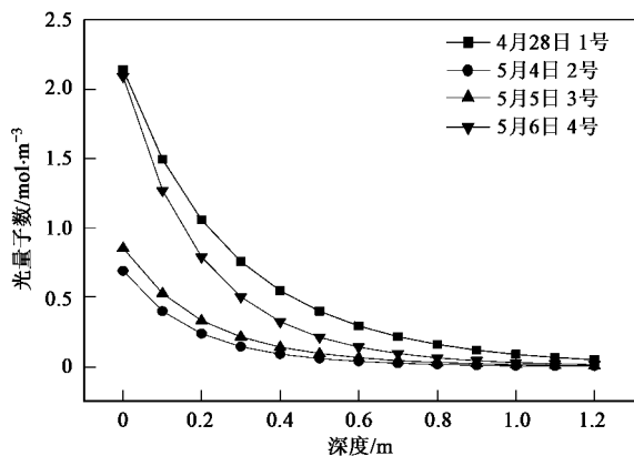
图4 各站点藻类吸收光量子数的廓线分布
