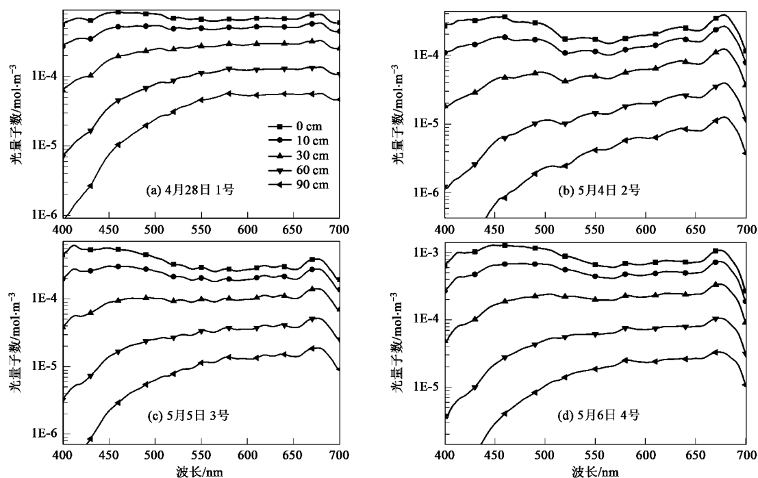
图3 不同站点藻类获取的光合有效辐射随深度的谱变化
