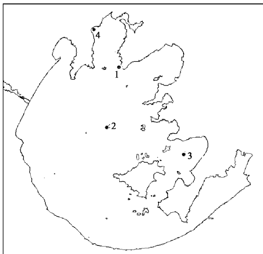
图 1 采样点分布示意
