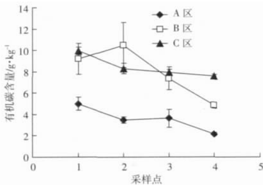
图 5 不同潮间湿地土壤有机碳变化趋势
