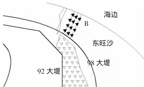
图3 B区样地采样示意图
