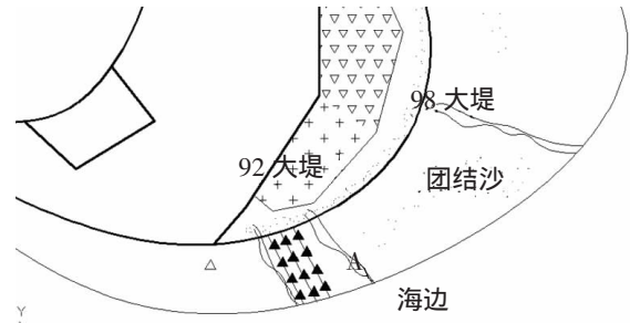
图2 A区样地采样示意图
