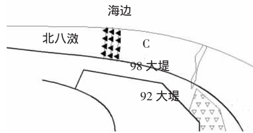
图4 C区样地采样示意图
