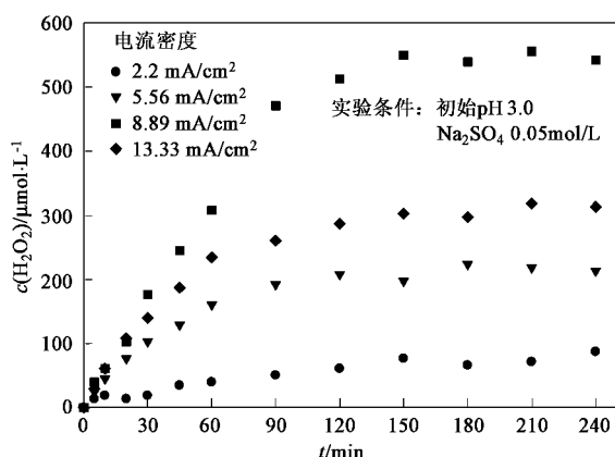
图 4 电流密度对 \text{H}_2\text{O}_2 产率的影响
