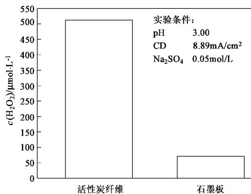
图 2 阴极材料对产 H 2 O 2 浓度的影响 (电解 240 min)
