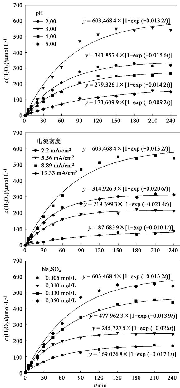
图 7 H 2 O 2 浓度与时间关系的拟合曲线
