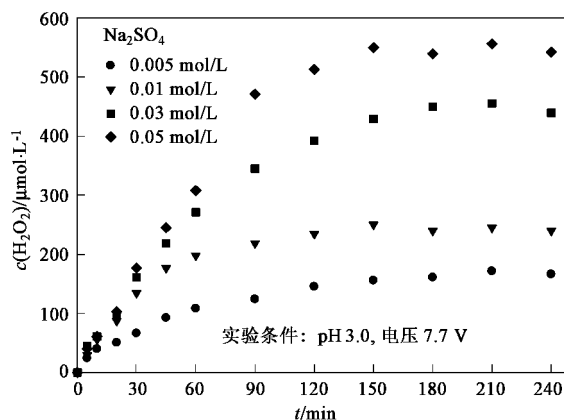
图 5 \text{Na}_2\text{SO}_4 浓度对 \text{H}_2\text{O}_2 产率的影响
