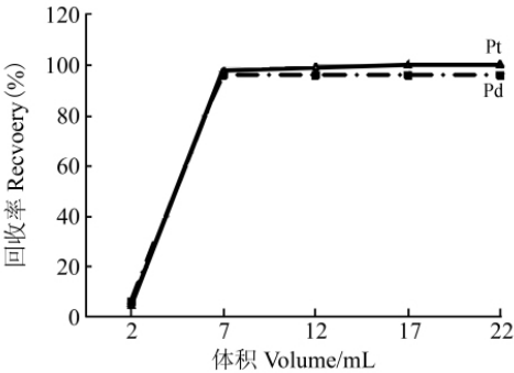
图 1 0.6 mol/L HCl 介质中主要 PGEs( Pt 和 Pd) 的回收率 Fig.1 Recovery of main platinum group elements ( Pt and Pd) in 0.6 mol/L HCl
