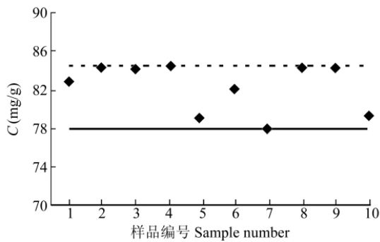
图3 国际标准物质 BCR-723 实验结果与标准值比较 Fig. 3 Comparison of Pt concentration in BCR-723 between experiment and certified reference values ◆: 实验值 ( Experimental value ) ; —: 标准值下限 ( Lower limit of standard vlaue ) ; ---: 标准值上限 ( Upper limit of standard vlaue ) 。
