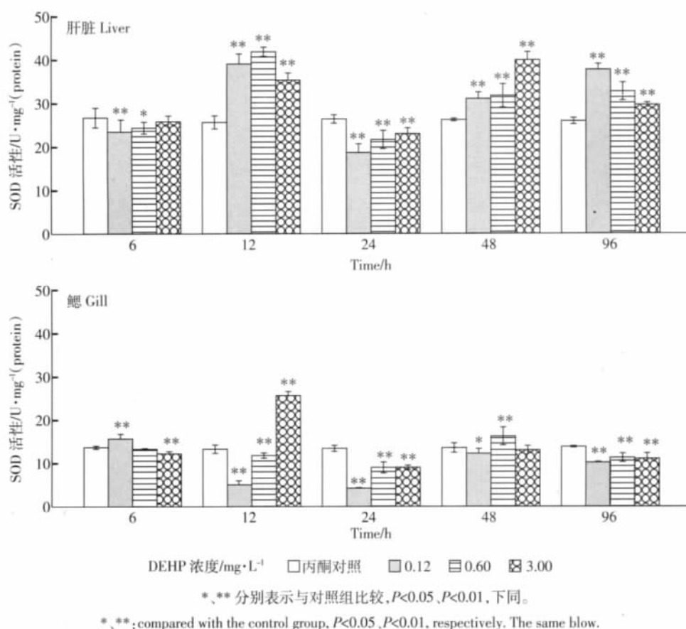
图1 DEHP对红鳍笛鲷肝脏、鳃组织SOD活性的影响
