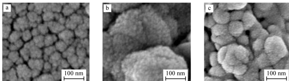
图 3 NiO( a) , Mb( b) 和 Mb/NiO/DMSO( c) 修饰在玻璃片上的扫描电镜图
