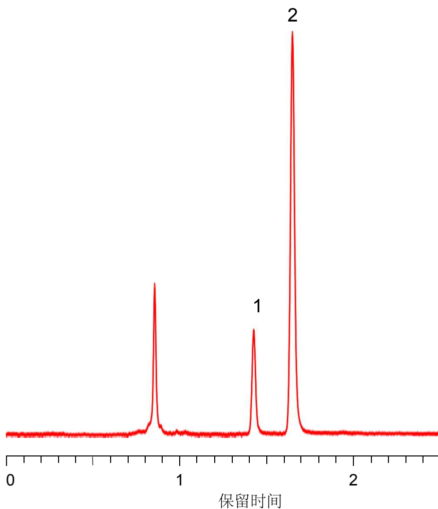
1. 三聚氰酸
