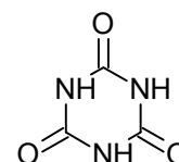
1. 三聚氰酸
