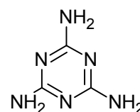
2. 三聚氰胺
