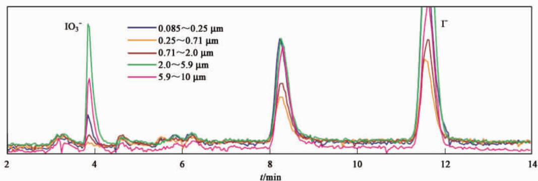
图3 IC-ICPMS 测定 Mace Head 地区气溶胶中碘形态色谱图 [62]
